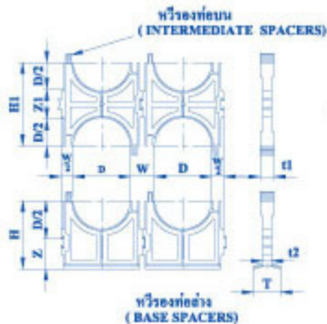
7.1 หัวรองท่อแบบ (INTERMEDIATE SPACERS)
